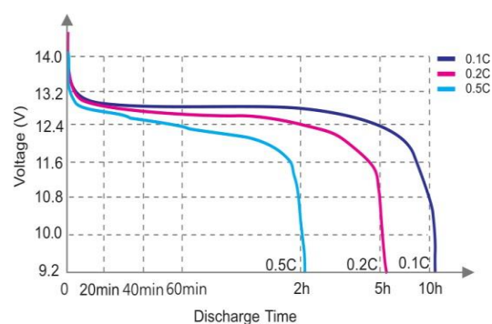
Courbes de décharge de différents courants
