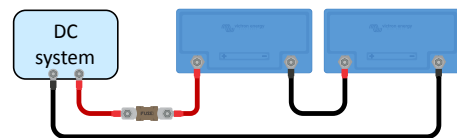
Connexion de plusieurs batteries en série
