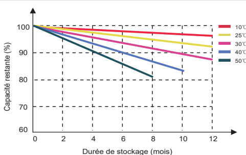
Courbe d'autodécharge à différentes températures
