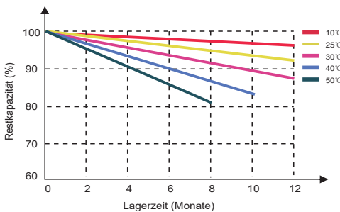
Unterschiedliche Temperatur-Selbstentladekurve
