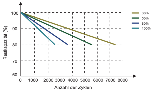
Unterschiedliche DOD-Entladungszyklus-Lebenskurve
