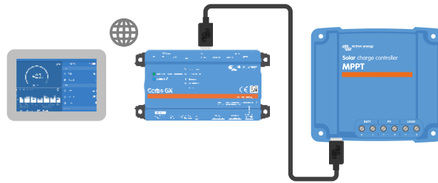
Connexion à l'application VictronConnect à travers le réseau LAN ou Internet (portail VRM) en utilisant un appareil GX (par exemple un Cerbo GX)
