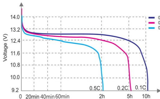
Courbes de décharge de différents courants
