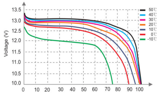
Courbes de décharge à différentes températures
